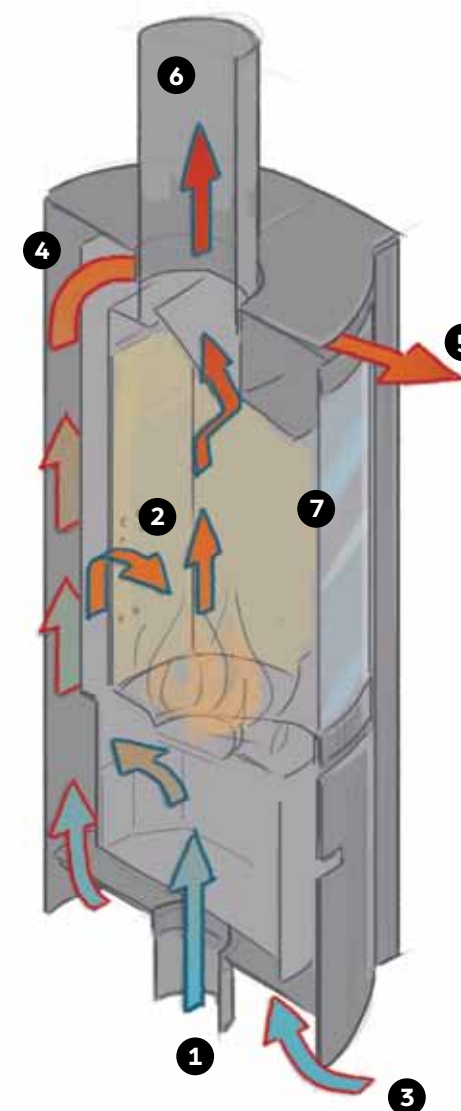
Tecnica di combustione e circolazione dell'aria Stûv 30-compact
